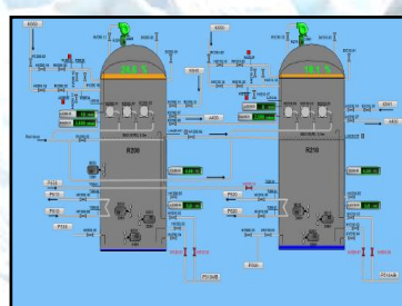
Digestores-Biogas
